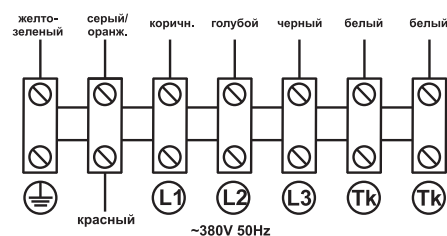
Схема подключения №4
